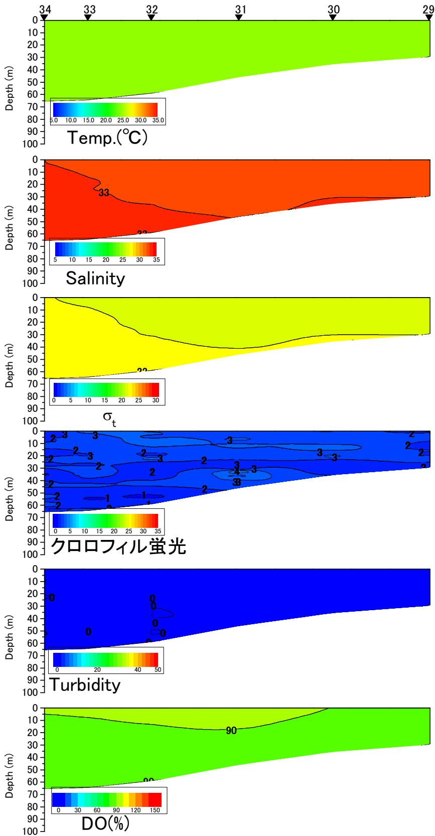
八代海西ラインの水温(°C)、塩分、密度( \sigma_t )、クロロフィル蛍光強度、濁度、溶存酸素飽和度(DO%)の鉛直面図(国土交通省の調査による) (2016年10月25日)
